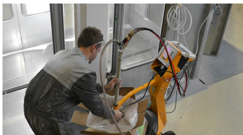
Krok 6: Włóż rurę ssącą do nowej farby
