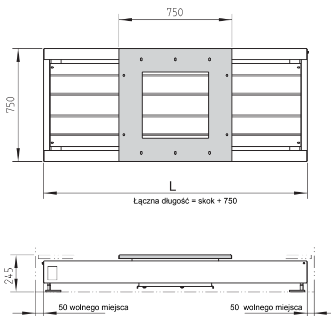
Oś pozioma YT04 - wymiary
