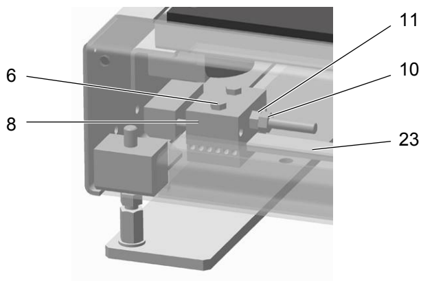
Oś pozioma YT04 – Naciąganie paska napędowego
