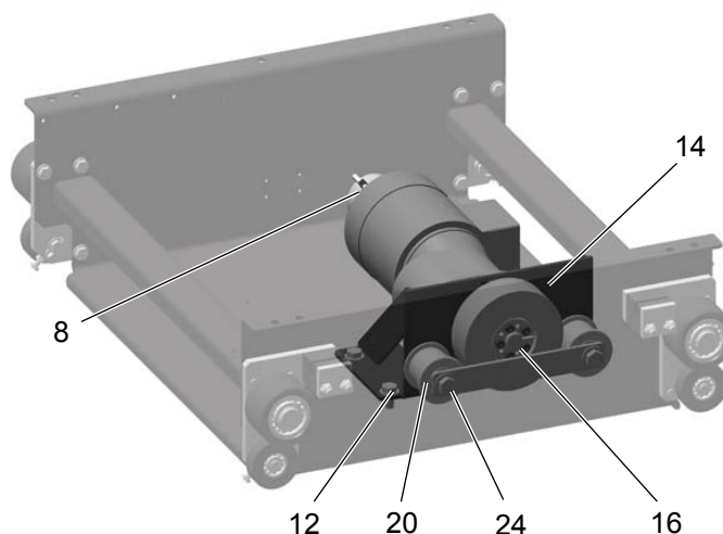
Oś pozioma YT04 - jednostka napędowa
