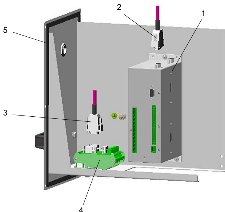
Oś pozioma YT04 - moduł elektryczny w manipulatorze ZA
