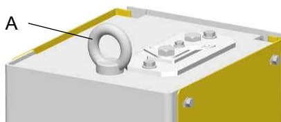
Manipulator ZA05 – widok z góry
